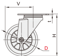
万向型 WHG01
