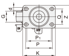
自由状态
