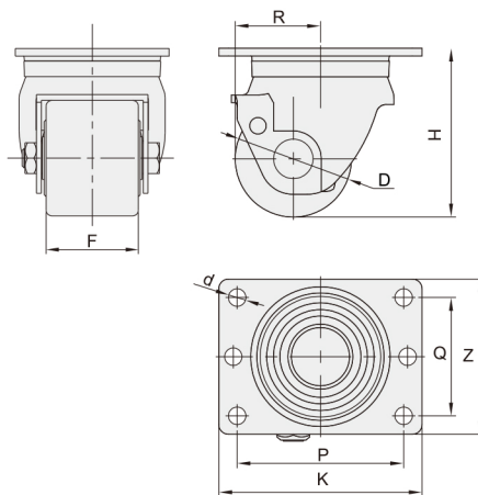
平底活动型 WKG52
