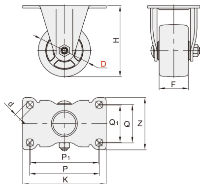
固定型 WKG41/42
