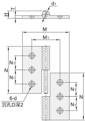
6孔安装
