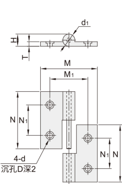
4孔安装
