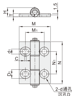
横向腰孔型 VKC43
