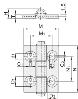
横竖向腰孔型 VKC45
