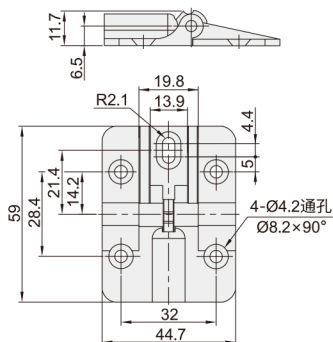
锥孔+腰孔型 VKR16
