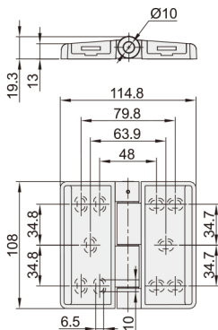
横竖向腰孔型 VKR12
