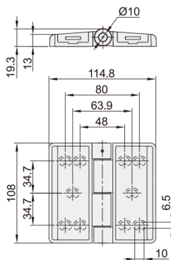
横竖向腰孔型 VKR13
