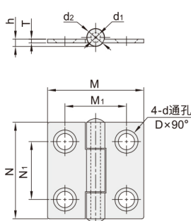
锥形型 VKJ05
