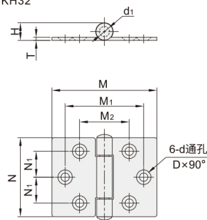
锥孔错位型 VKH32
