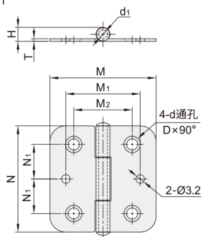
锥孔带定位孔型 VKH31
