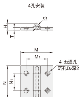
沉孔型 VKH34
