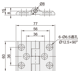
锥孔错位型 VKH33
