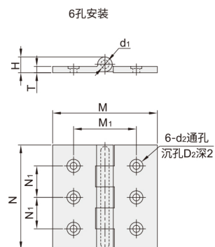
沉孔型 VKH34
