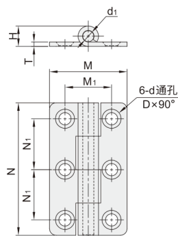
VKH16 6孔安装
