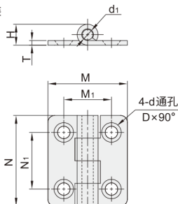
VKH16 4孔安装
