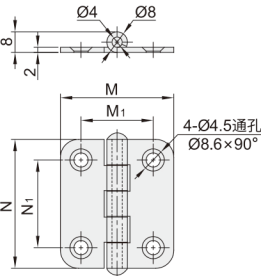
VKH16 4孔安装
