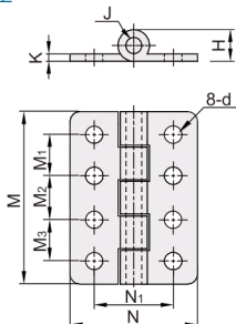
沉孔型 A型
