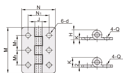
沉孔型 B型
