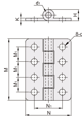
C形安装
