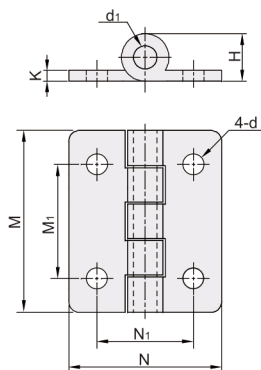
A形安装
