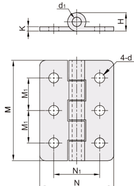
B形安装
