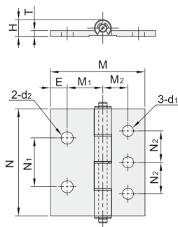
圆孔型 VKC46
