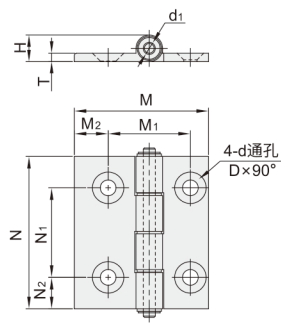
锥孔型 VKC48
