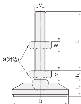
全尼龙底座型 WBS11 D=50/80
