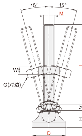
全金属底座型 WBS12/13
