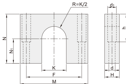
薄壁型 WAF06
