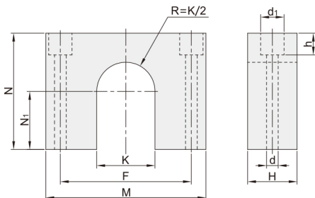
标准型 WAF05
