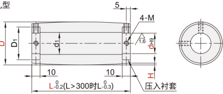
带肋槽直柱型 VBF21/26/31 圆孔+螺孔型
