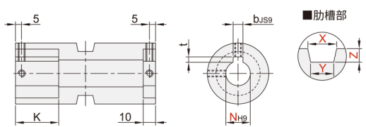
键槽孔+螺孔型
