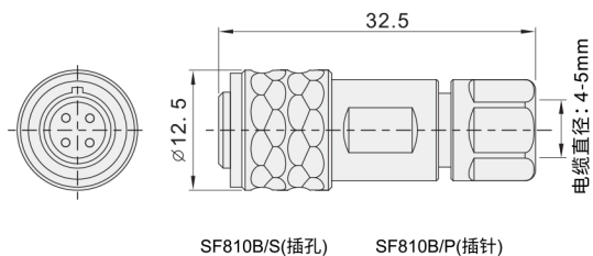
电缆插头
