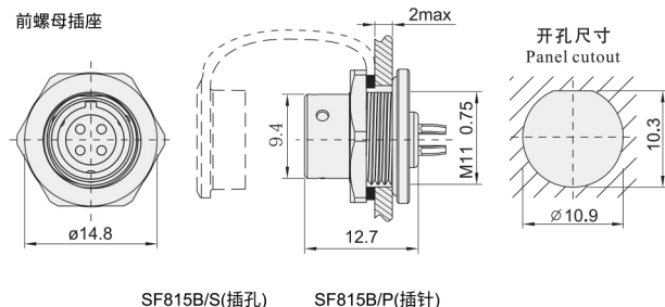
SF815B/S(插孔)
