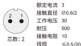
公端绝缘体正面图
