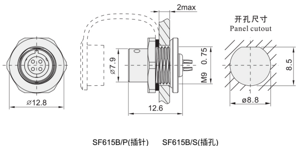
前螺母插座
