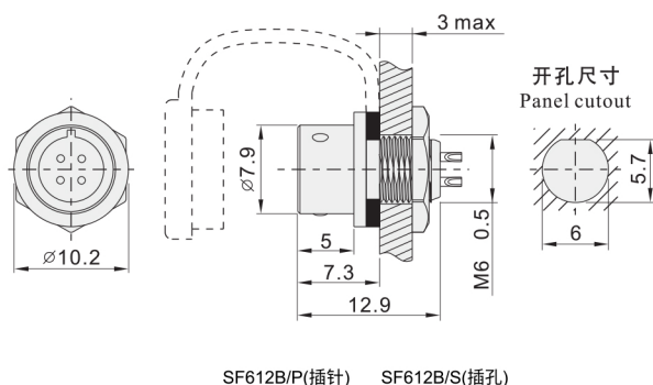
后螺母插座
