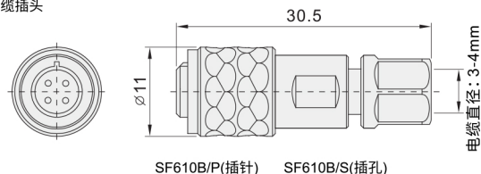
电缆插头
