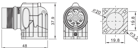
ZL 公针弯式方形法兰插座
