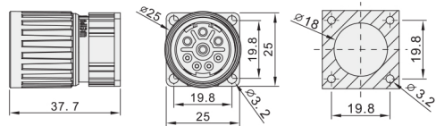
Z 母针直式方形法兰插座
