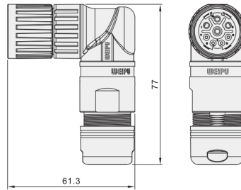
TL 母针 弯式电缆插头
