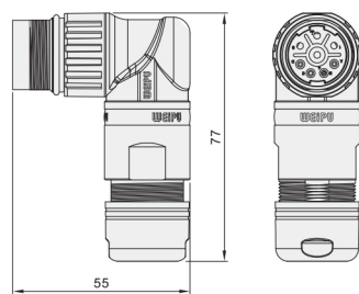
TL 公针 弯式电缆插头
