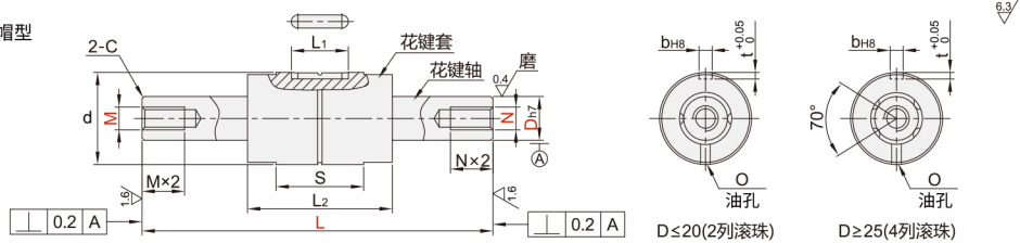
圆法兰螺母型 HLT36
