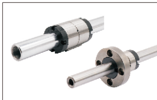
圆筒螺母型 HLF31
