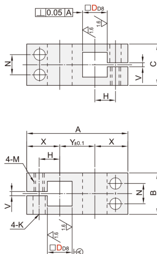
方孔+方孔 ODD41/42/51/52/61
