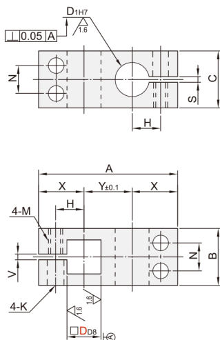
方孔+圆孔 ODD01/02/11/12/21
