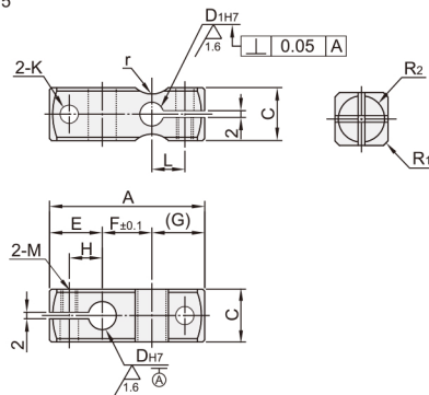
异径正交 ODC41/42/51/52 D8~15
