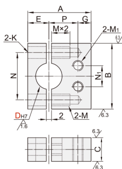
螺纹垂直型 OED01/02
