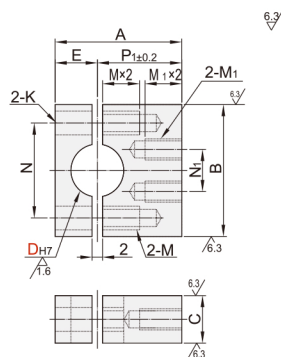
螺纹平行型 OED11/12
