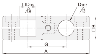
组合体
