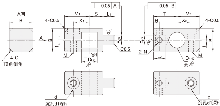
组合体
