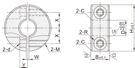
紧凑型 SBQ01/02/06
