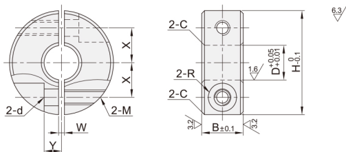
平衡型 SBQ51/52/56
