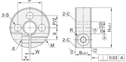
三孔锁紧型 SBL01/02/06
