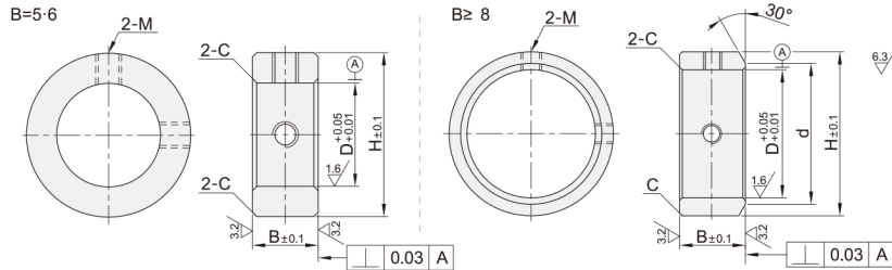
双孔型 SBC41/42/46
