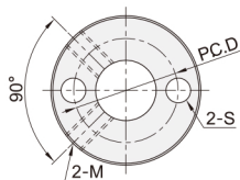
双孔型 SBC41/42/46
