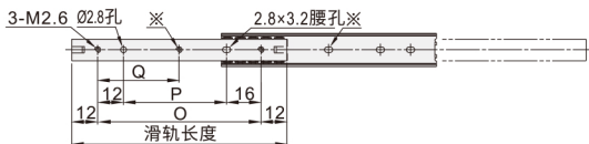
两段式.3/4伸展 VZP53
