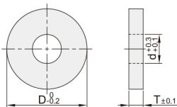
垫圈 SAA41
