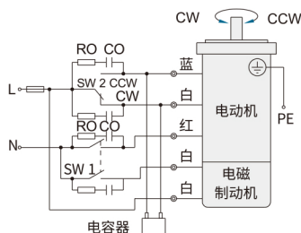
■ 接线示意图 15W,1ph110V
