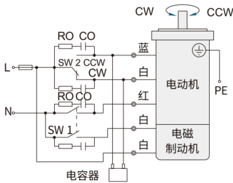
■ 接线示意图 6W,1ph110V
