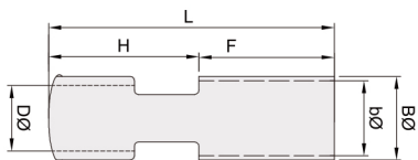
子弹型绝缘对接端子 DZB11
