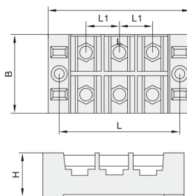
TB固定式端子排 OTD41
