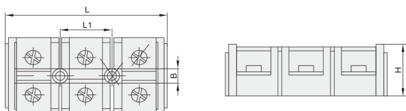
TBR/TC大电流端子排 OTC91
