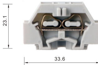
262-301-307 厚度:7mm
