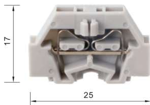
260-301-307 厚度:5mm
