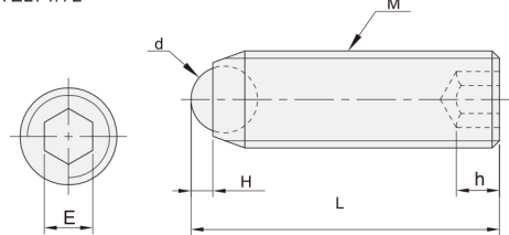
紧定螺钉型 YZL71/72
