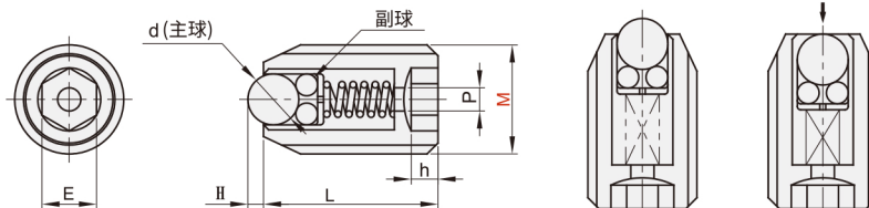
滚珠型 YZL41/42
