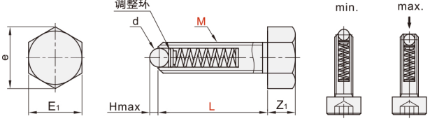
外六角螺栓型 YZK11 YZK12
