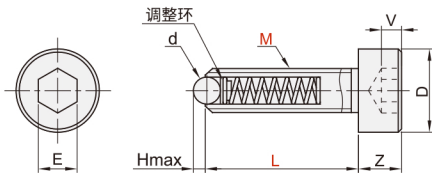
内六角螺栓型 YZK01 YZK02
