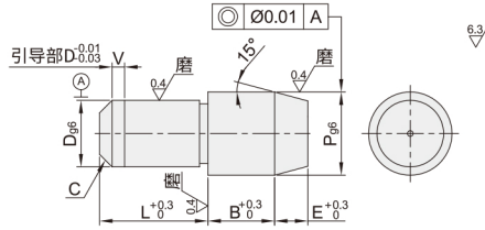
■ P尺寸公差表
