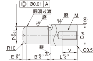
内螺纹型 MEH10/11/12/13
