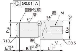
内螺纹型 MEH14
