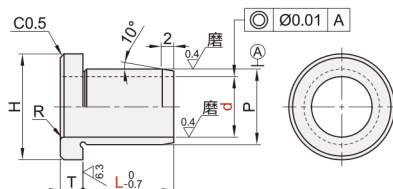
带肩型·薄壁型 MEF21/22/23/31/32/33
