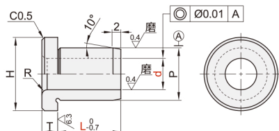
带肩型·标准型 MEF01/02/03/11/12/13
