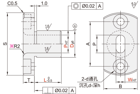
对边法兰型 MEB21/22
