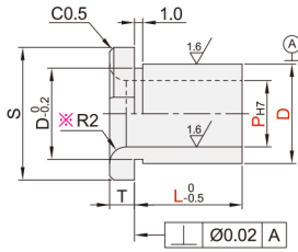
带肩型 MEB01/02/11/12
