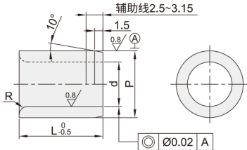
无肩型 MER01
