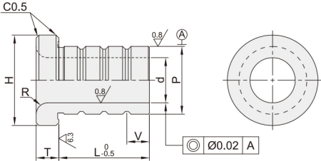
带肩型 MER12
