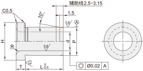
带肩型 MER12
