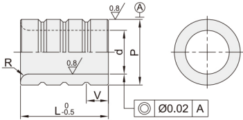
无肩型 MER11
