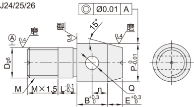
圆型 MEJ21/22/23 MEJ24/25/26
