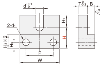
侧面安装型-L型 ACC11/12/20
