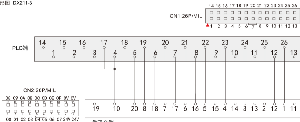
外形图 DX211-3
