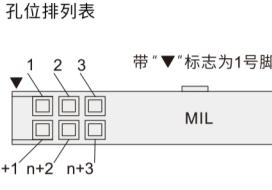
孔位排列表
