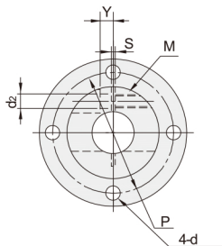
开口法兰型·圆法兰型 ZRJ01/02/03
