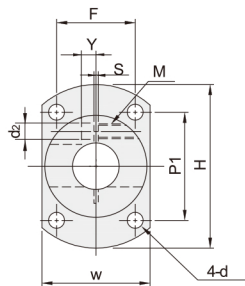
开口法兰型·两面切割法兰型 ZRJ31/32/33
