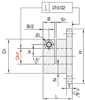
开口法兰型·方法兰型 ZRJ21/22/23
