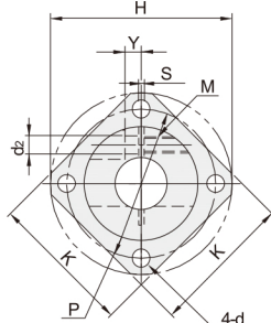
开口法兰型·方法兰型 ZRJ21/22/23
