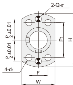
定位孔螺孔型·两面切割法兰型 ZPU31/32/33
