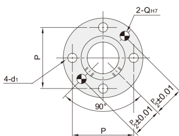
定位孔螺孔型·圆法兰型 ZPU01/02/03
