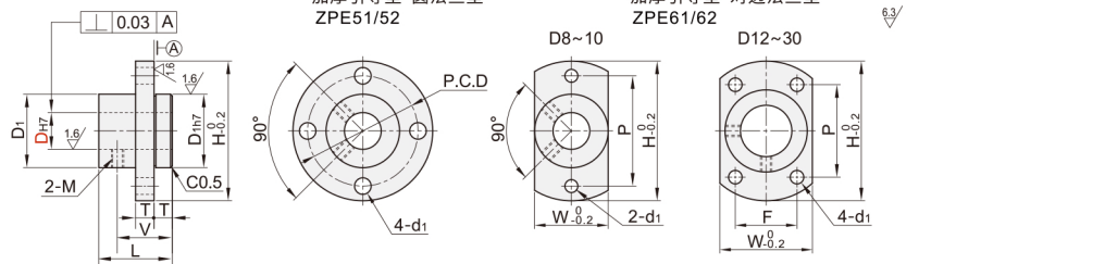
加厚引导型·圆法兰型 ZPE51/52
