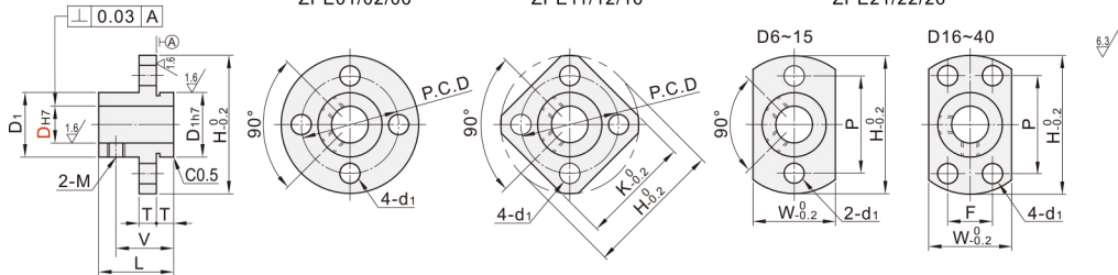
加厚引导型·圆法兰型 ZPE51/52
