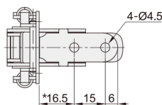
HAR42 垂直安装
