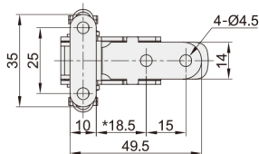
HAR41 平行安装
