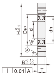
无扣环型
